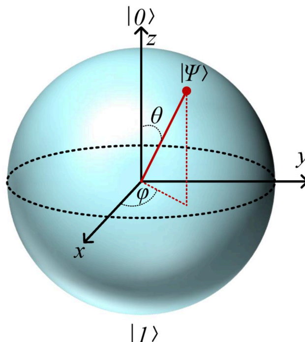
Visualization of the state of a qubit \Psi in the Bloch sphere 「ブロッホ球におけるキュービット \Psi の状態可視化」
